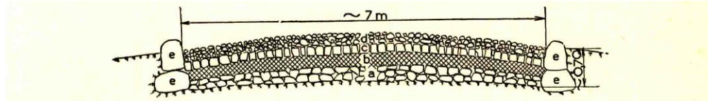
Fig. 1.01.01. Oud-Romeinse weg; a = bed van grote onregelmatige stenen; b = dikke laag beton (Romeinse cement); c = laag keien; d = laag onregelmatige stenen met zand (ingereden door het zware verkeer); e = kantstenen.
